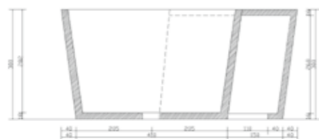
Schnitt 1-1
